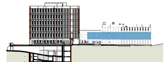
Ansicht Südfassade
